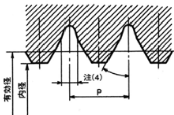
図一 3 切り取ったフランクを持つ山形 (ねじリングゲージに適用)
