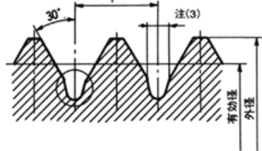
図一 2 完全なフランクを持つ山形 (ねじプラグゲージに適用)
