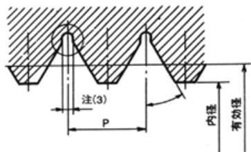
図一 1 完全なフランクを持つ山形 (ねじリングゲージに適用)
