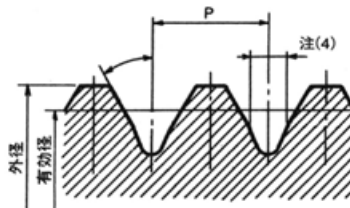
図一 4 切り取ったフランクを持つ山形 (ねじプラグゲージに適用)
